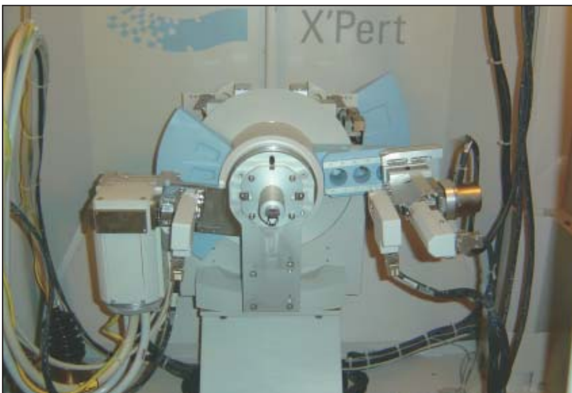
Goniometer
